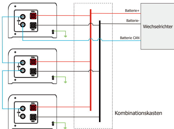
Abb. 4-1 Parallelschaltung von drei Batterien
