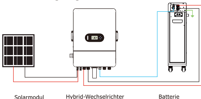
Abb. 3-1 Anschlussdiagramm für ein Einzelbatteriesystem
