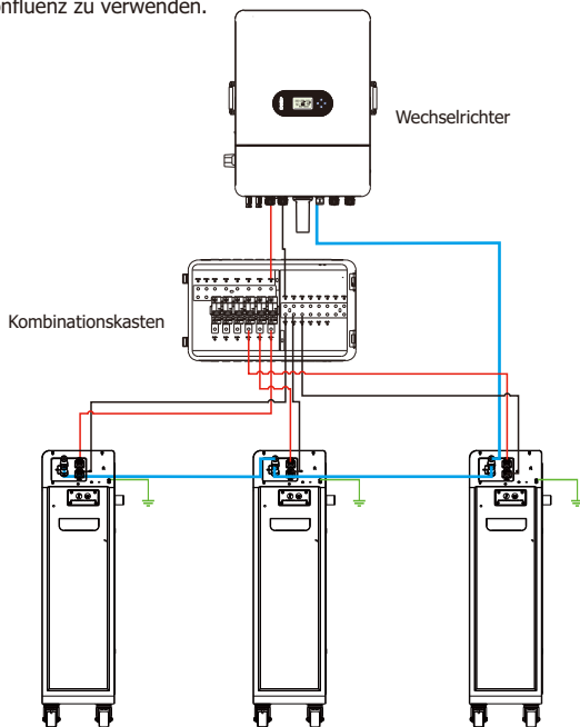
Abb. 4-1 Parallelschaltung von drei Batterien
