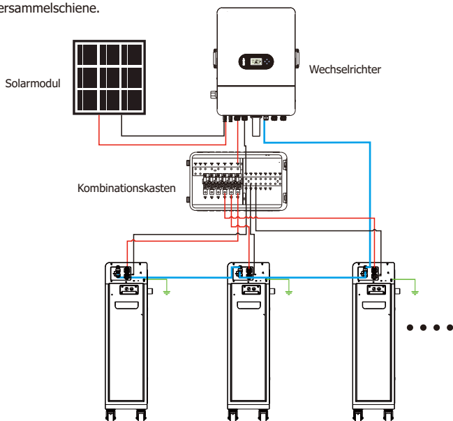
Abb. 3-2 Anschlusschema für ein Parallelsystem mit mehreren Batterien
